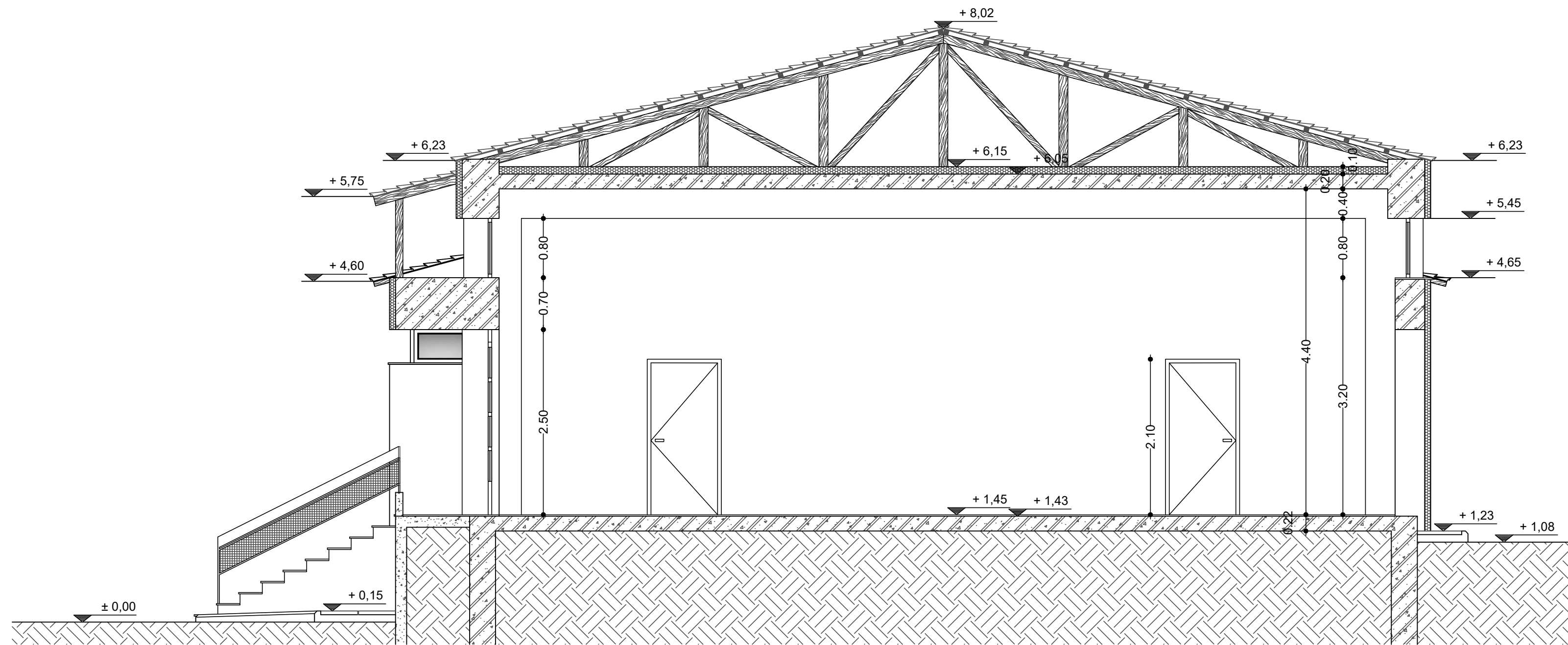
ΤΟΜΗ Β-Β
