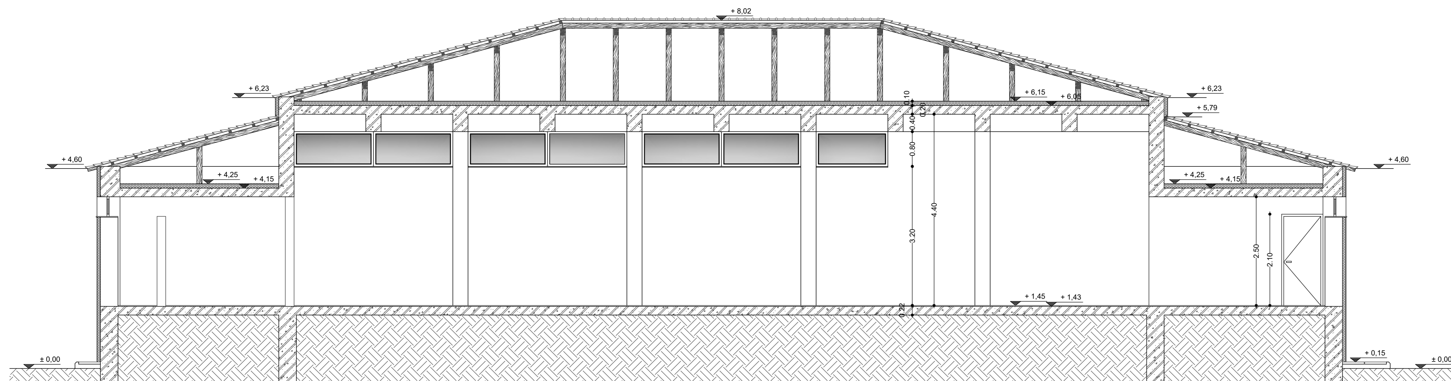
ΤΟΜΗ Α-Α
