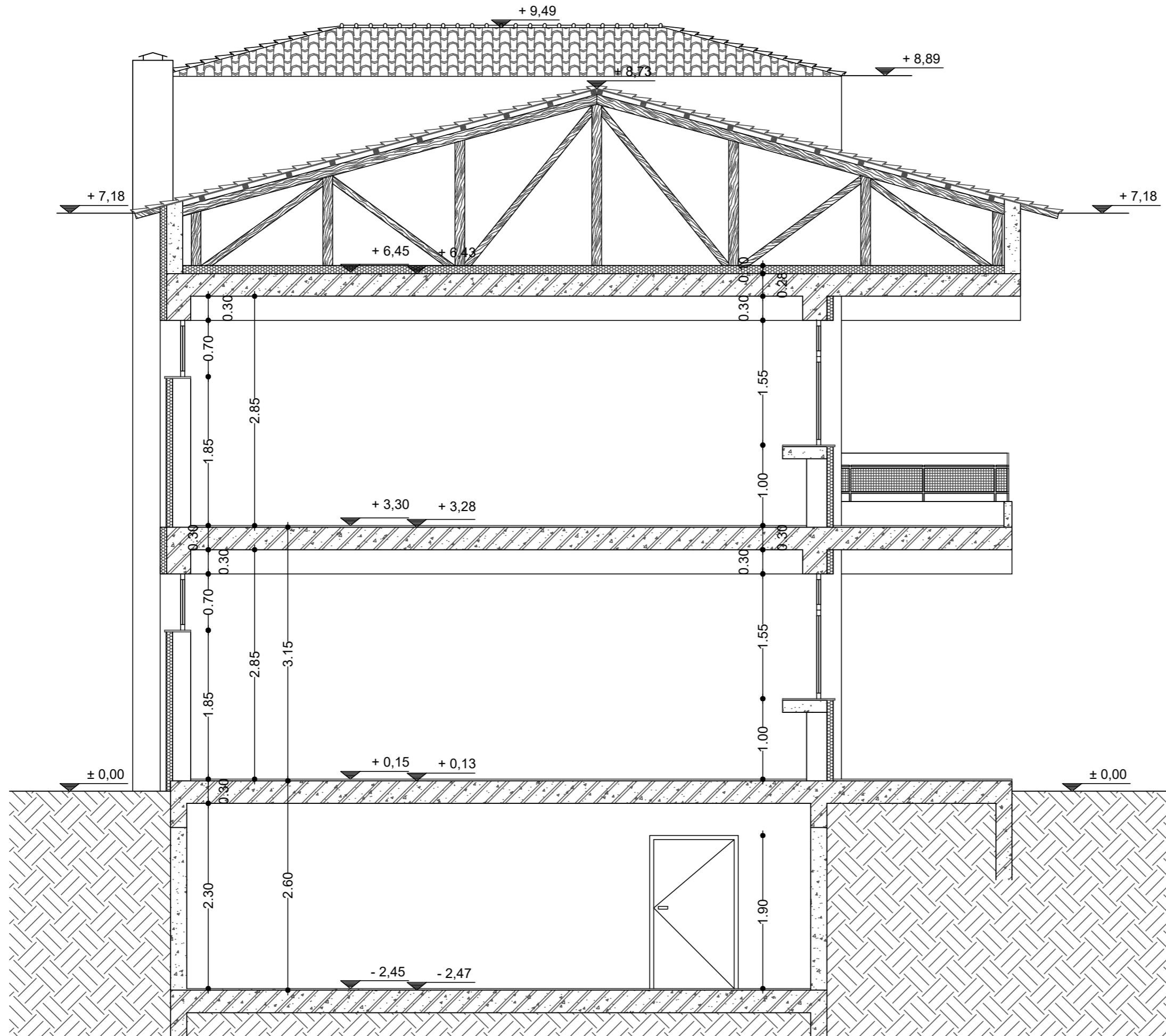
ΤΟΜΗ Β-Β
