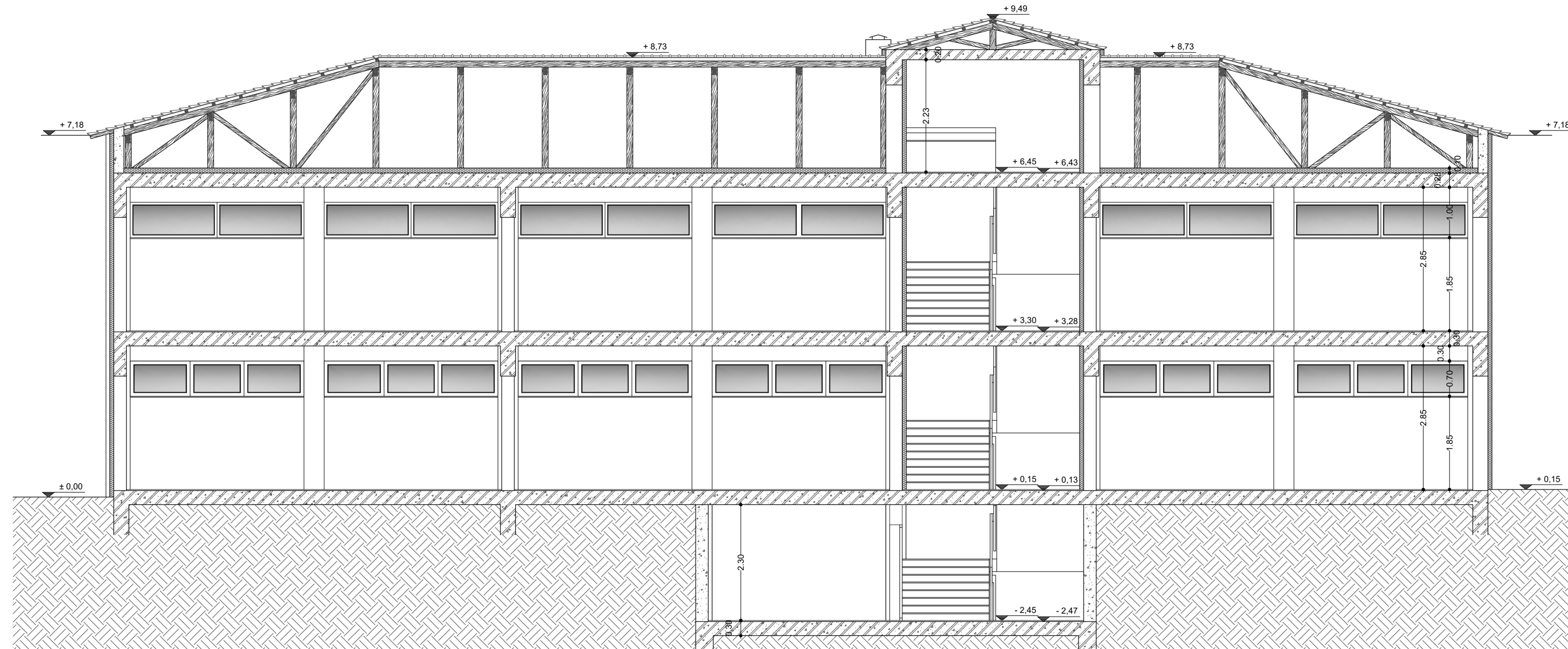
ΤΟΜΗ Α-Α
