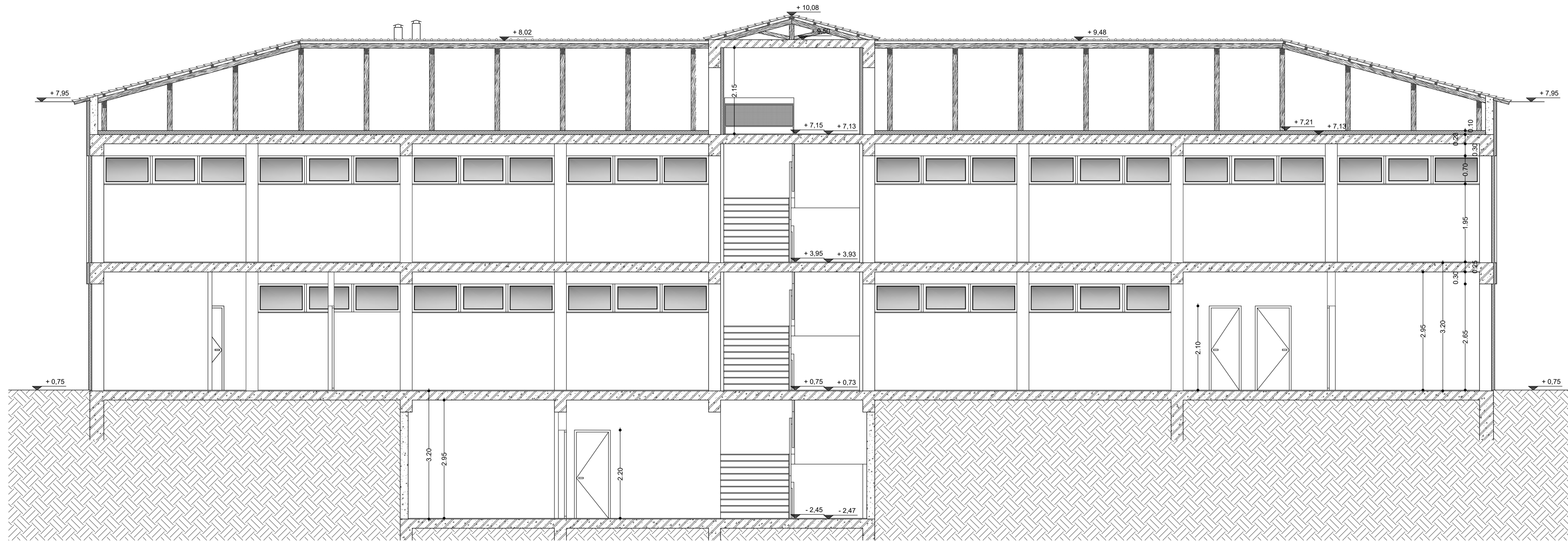
ΤΟΜΗ Α-Α
