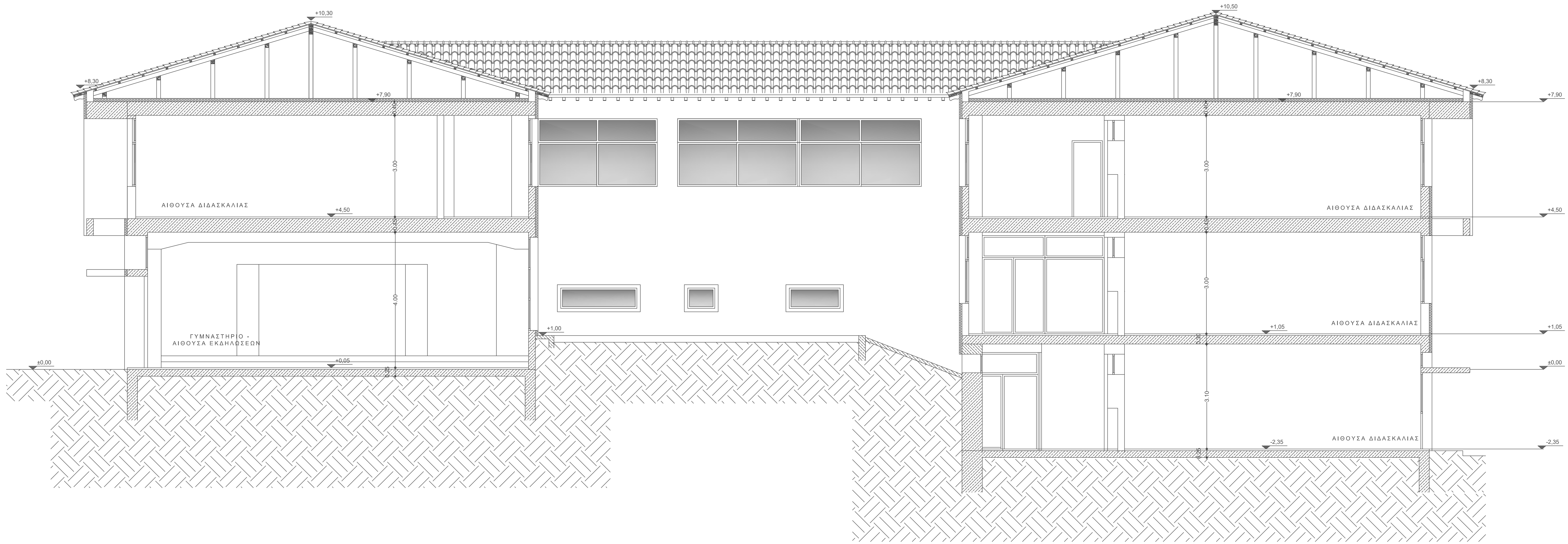
ΤΟΜΗ Β - Β
